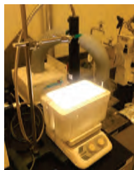
ソーラーシミュレーターによる環境汚染物質の光化学反応試験
