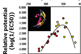
環境汚染物質のダイオキシン受容体活性化能に対する構造活性相関解析
