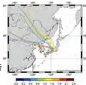
気塊の流跡線解析
